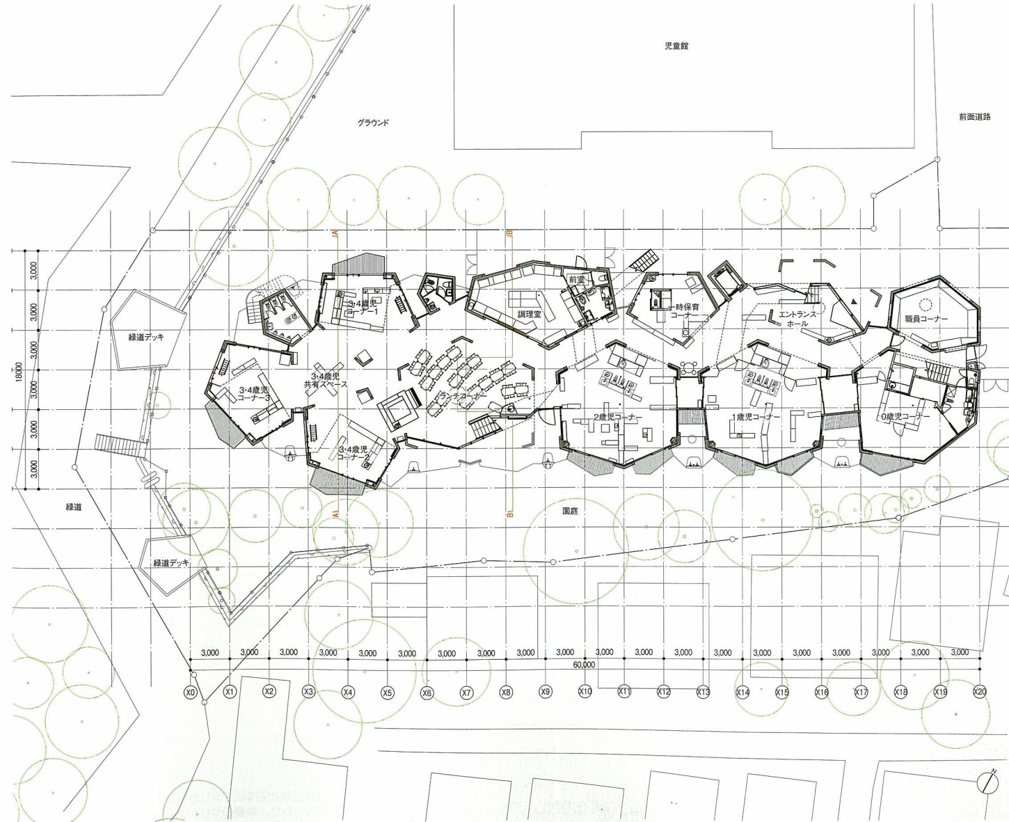
1階平面 縮尺1/400
